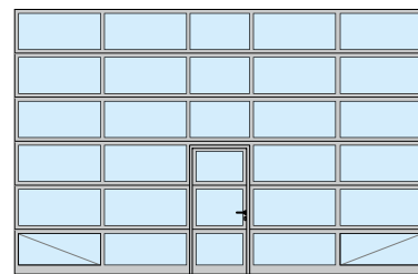
ALR F42, ALR F42 Thermo, ALR 67 Thermo разположение на вградената врата в средата цялостно остъкление
