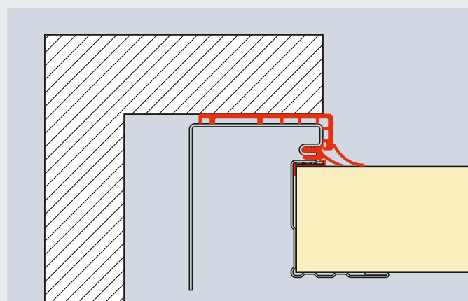
Страничен ограничител с ThermoFrame
