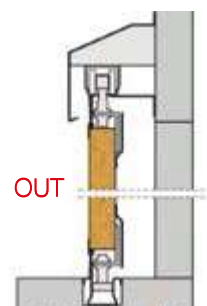
Hanging with floor track Suspendue avec rail au sol Suspendida con guía de tierra
