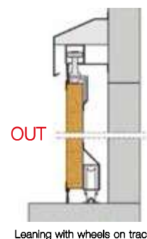
Leaning with wheels on track Soutenu avec roulettes dans le rail Apoyado con ruedas sobre guía
