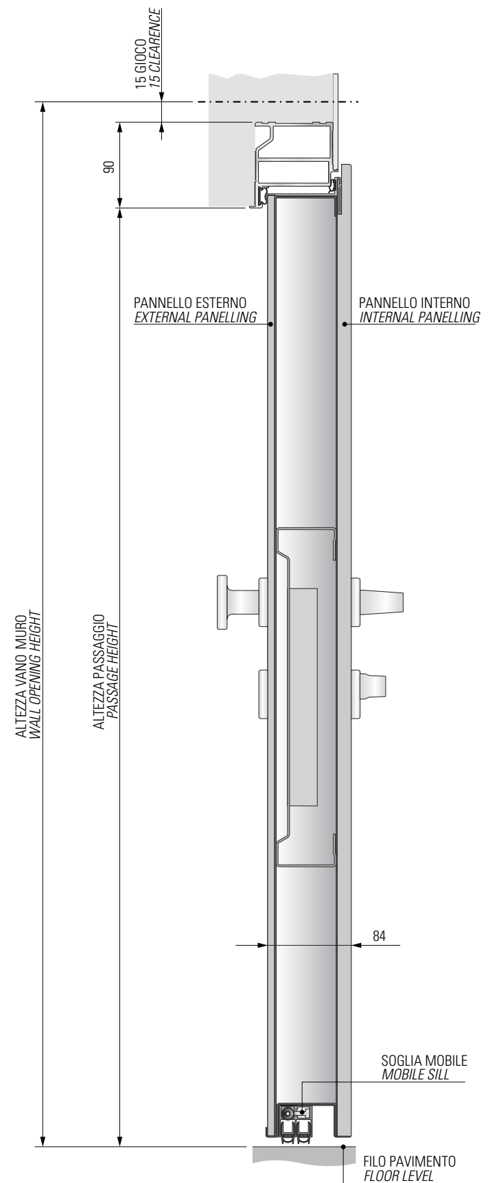
SEZIONE VERTICALE VERTICAL SECTION
