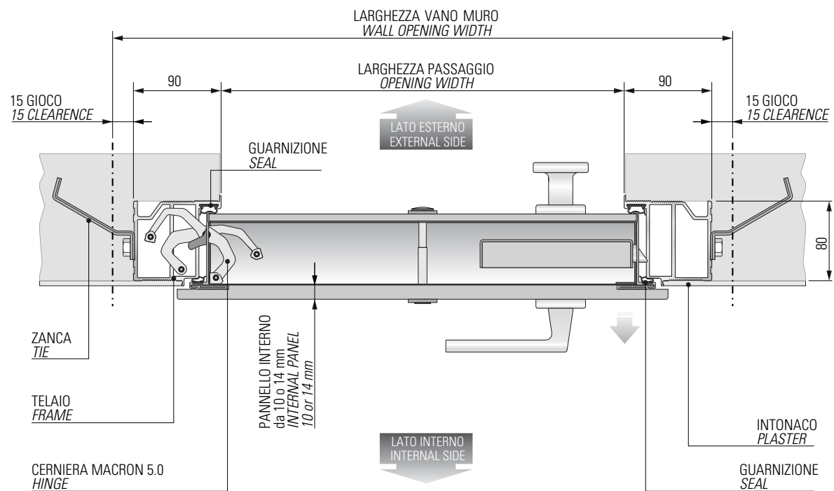
SEZIONE ORIZZONTALE HORIZONTAL SECTION
